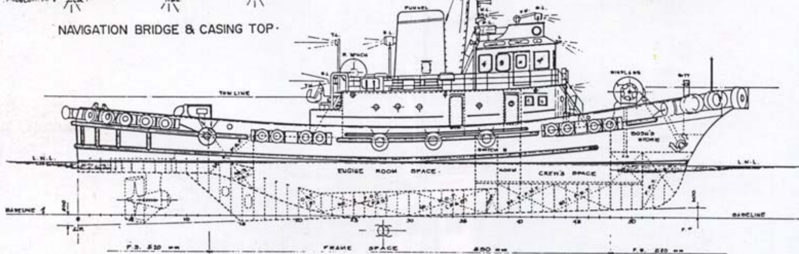
· OUTBOARD PROFILE ·
